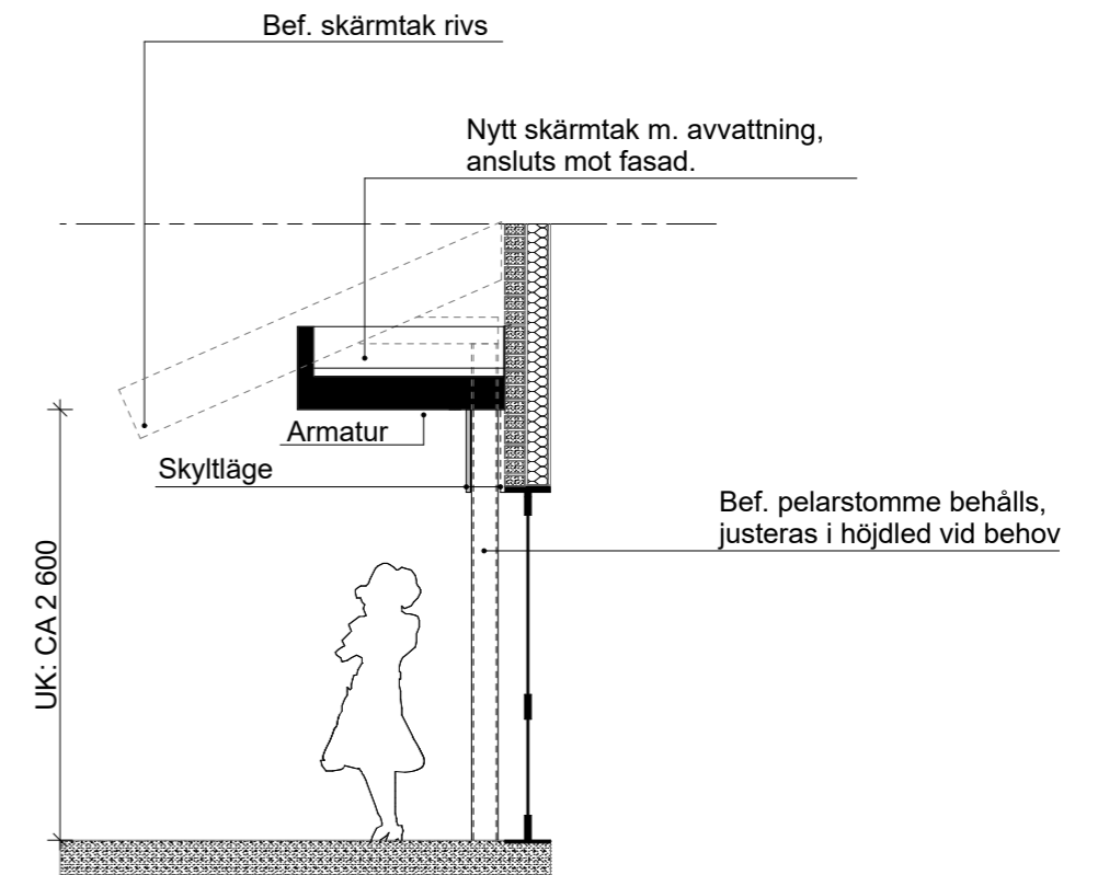
Pricipsektion skärmtak
